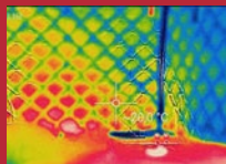
Aufnahme im Hochdach. Innen 20 °C, Außen -20 °C.
