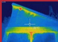
Aufnahme bei -20 °C mit BlidimaX® und BlidimaX®roof.
